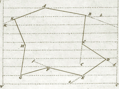
Fig. 34 Plain Table
